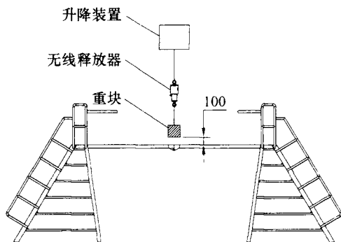
图 8 动载荷试验布置示意图
