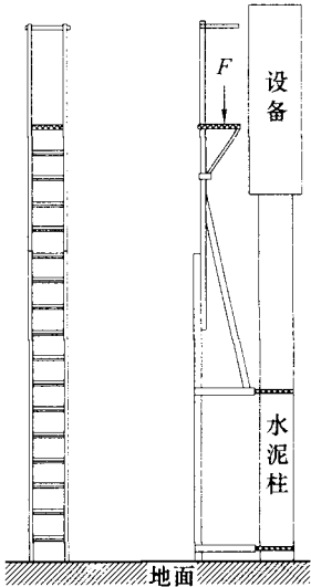
b) 伸缩型抱杆梯
